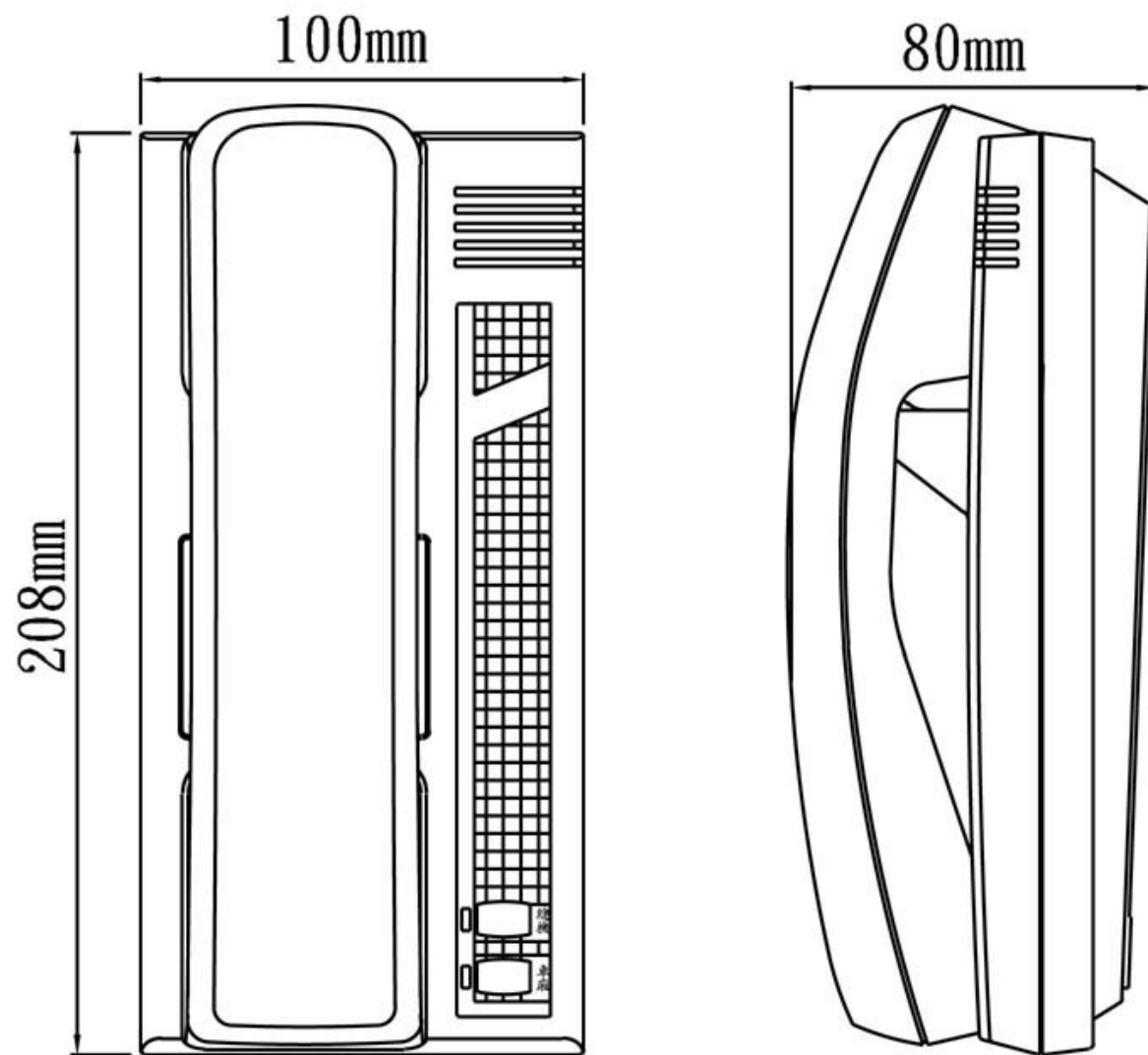
CT-701 數位電梯親機
